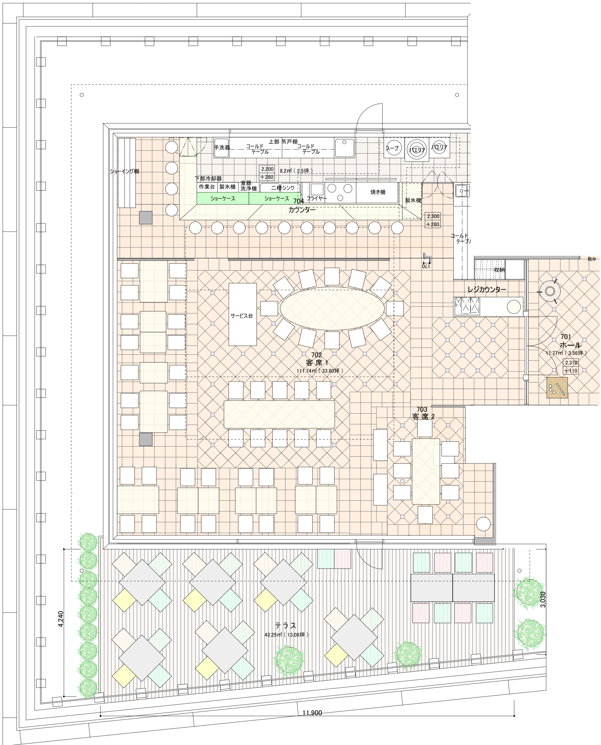
テラス平面図 1:50
