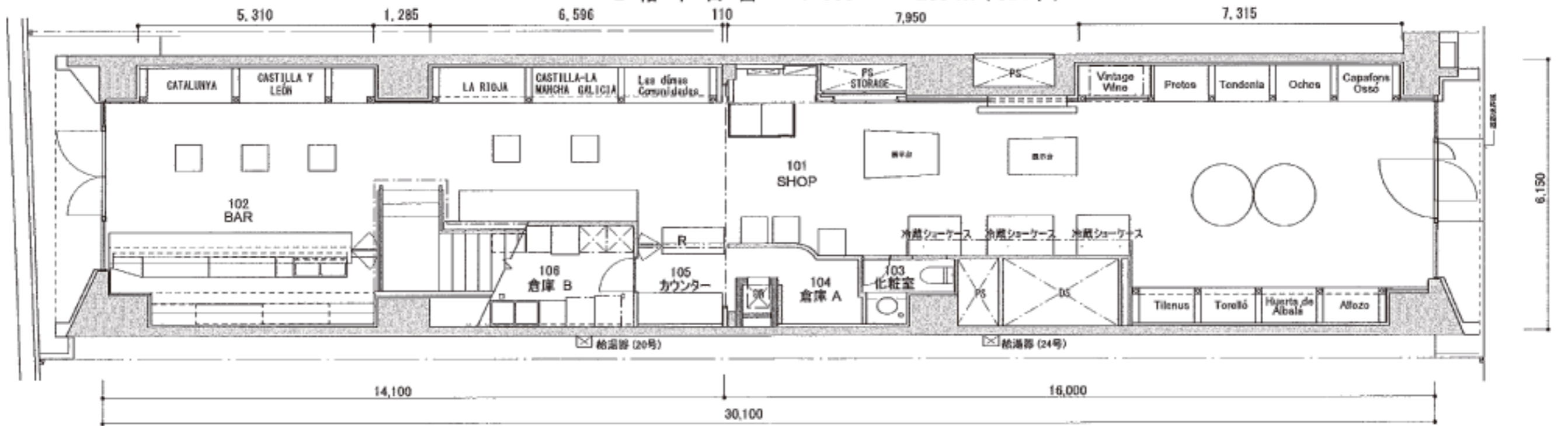
1階平面図 1:100 191㎡(58坪)
