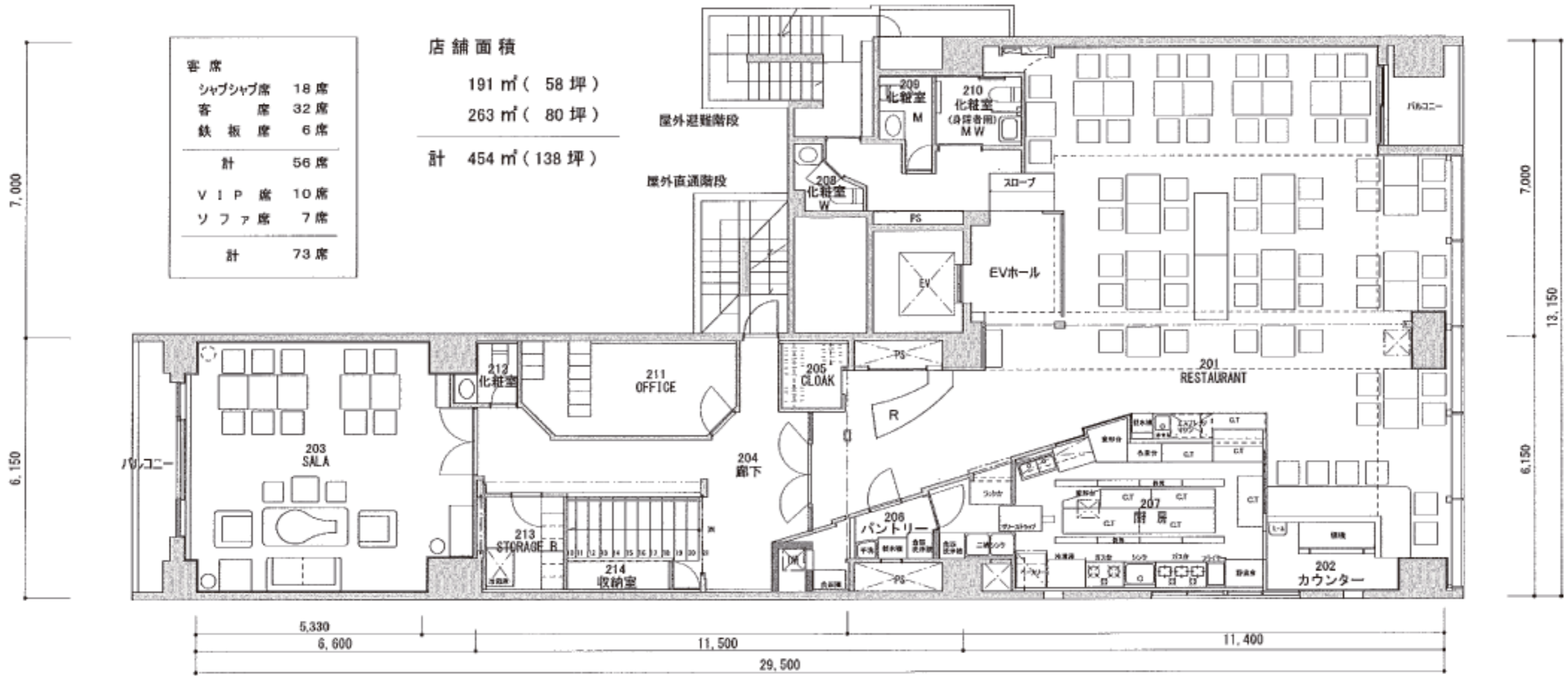
2階平面図 1:100 263㎡(80坪)
